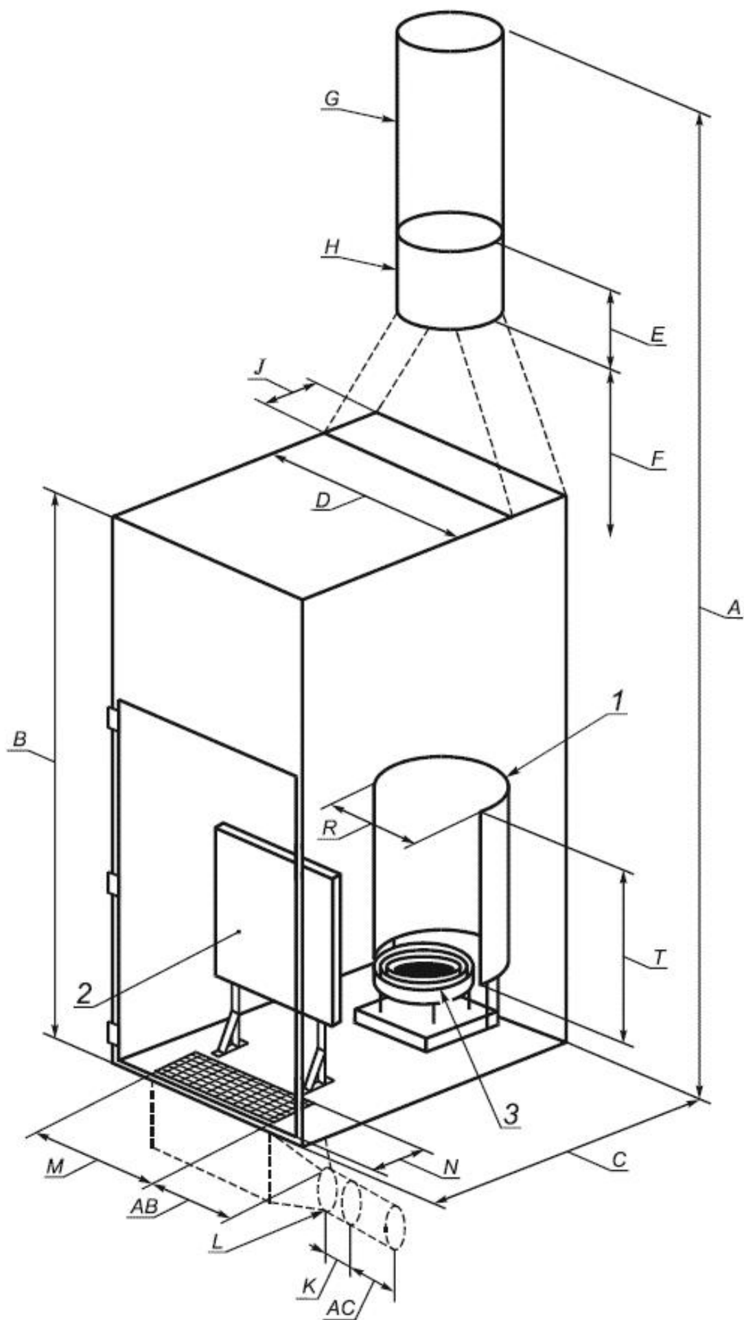
1 - экран; 2 - радиаторная панель; 3 - сосуд со спиртом
