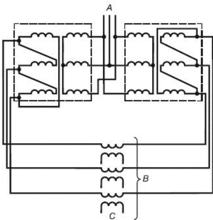
Рисунок ДВ.2 - Пример метода взаимной нагрузки - трехфазная схема
