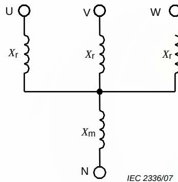
Figure C.1 – Schéma équivalent d'une bobine d'induction triphasée comprenant le couplage magnétique entre phases
