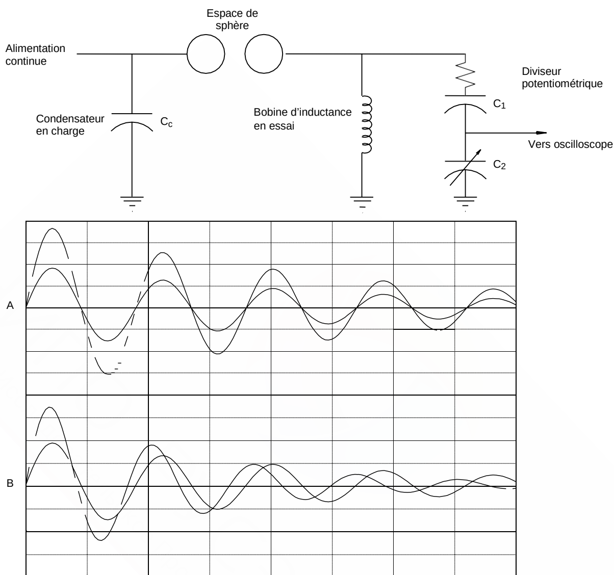
Figure E.1 – Circuit d'essai pour essai de surtension entre spires et oscillogrammes d'échantillon
