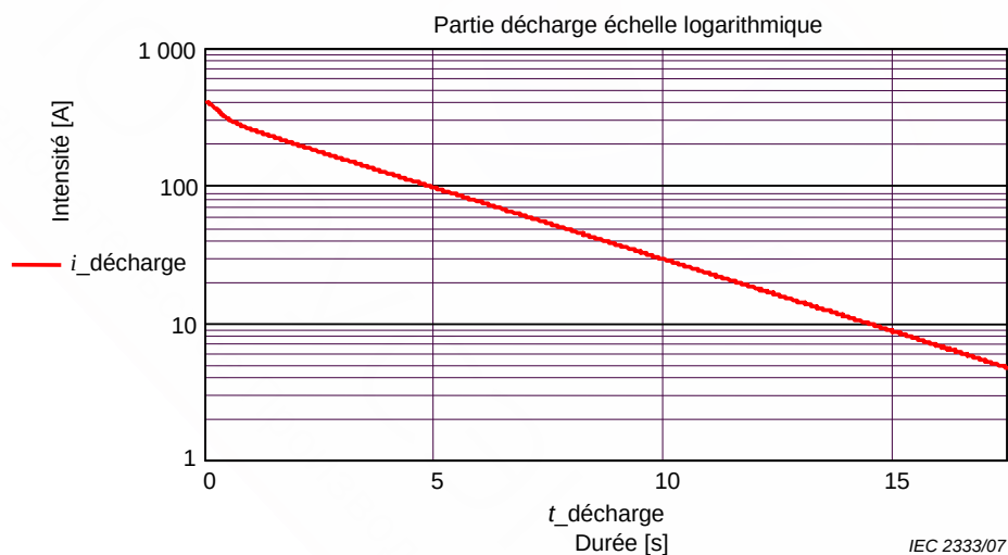
Figure B.4a – Graphique du courant de charge et décharge
