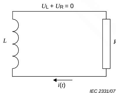
Figure B.3 – Circuit équivalent avec la bobine d'inductance court-circuitée
