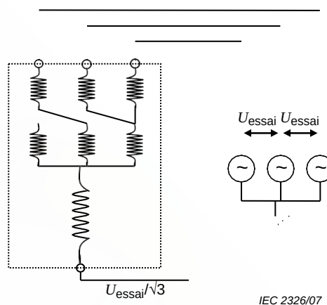
Figure 9 – Circuit d'essai de défaut monophasé avec alimentation de tension à la terre
